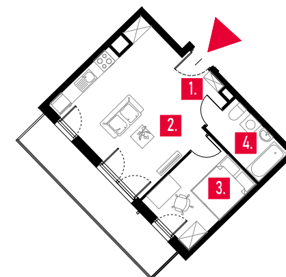
Rzut lokalu
