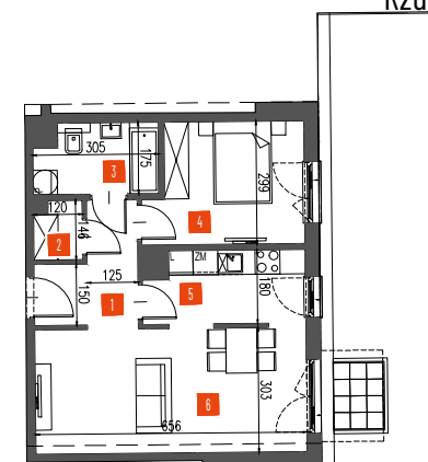
Rzut lokalu
