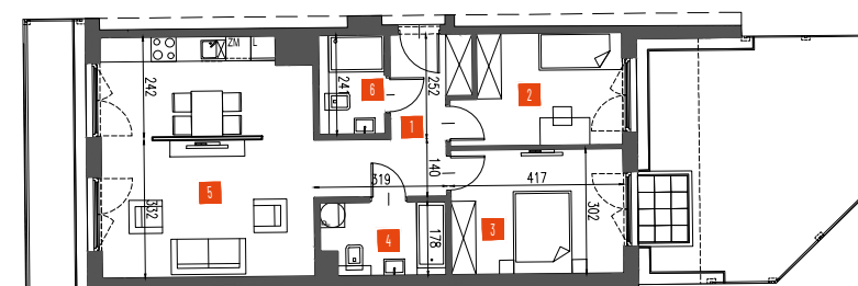
Rzut lokalu
