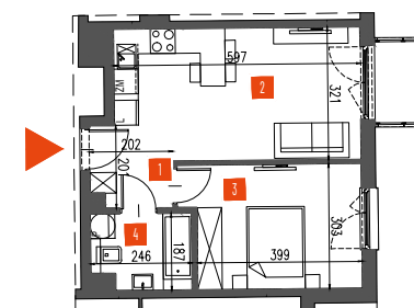
Rzut lokalu
